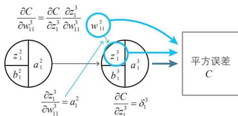
例3 的变量关系图。 神经单元等遵循 3-1 节的表示方法。
