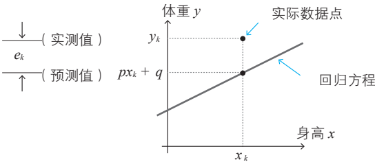
用图说明式 (3) 和式 (4) 的关系。第 k 个学生的 x_k 、 y_k 、 e_k 的关系图。
